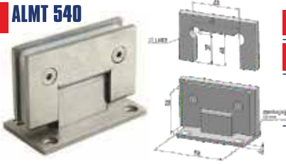
Cam Duvar Paraduş Menteşe Glass To Wall Paradus Hinge
