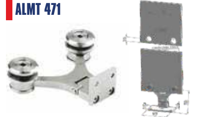
Cam Duvar Spider Yaysız Menteşe Glass To Wall Spider Unsprung Hinge
