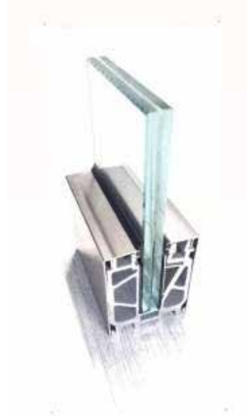
S Serisi 8-10-12-16-20mm Cama Göre Baza Kütük 15-30cm
