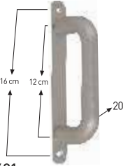
• 1601 Aynalı Çekme Kol Pull handle with rozette
